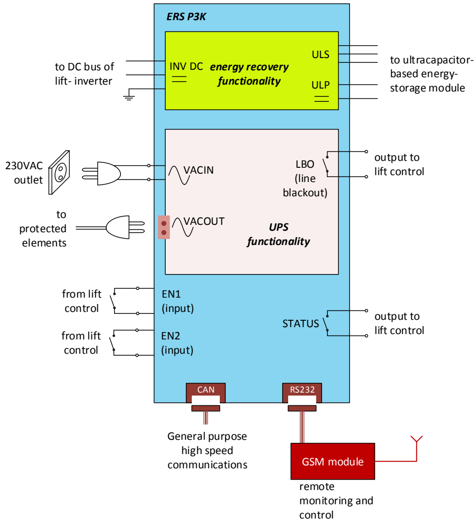
Fig. 2. ERS+UPS device
